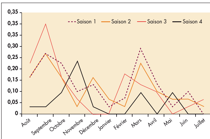
FIG. 14.– Variations mensuelles de la fréquentation de la source ferrugineuse par les Gypaètes barbus: détail par cycle annuel (n visites/n jours de suivi, septembre 2018; n = 145 ).
