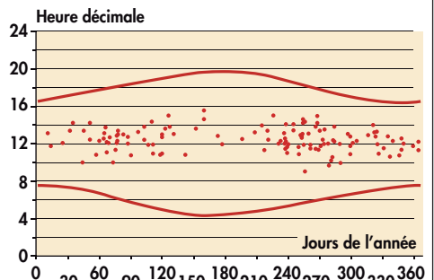
FIG. 4. – Fréquentation de la source ferrugineuse par les Gypaètes barbuis : données horaires en fonction du cycle saisonnier (en Temps Universel). Chaque point représente une visite ( n = 120 ); les courbes indiquent les heures de lever et de coucher du soleil; 0 = 1 er janvier.
