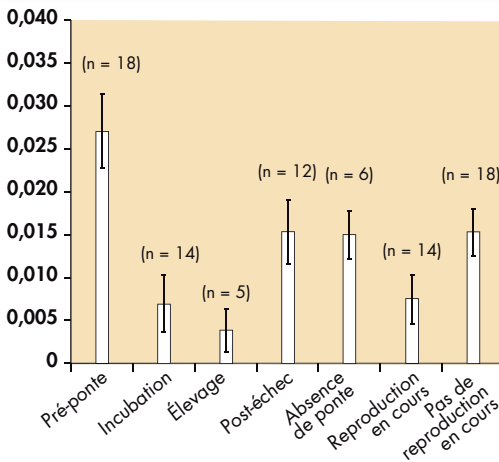
FIG. 16. – Fréquence des visites à la source ferrugineuse en fonction du stade de la reproduction chez 8 Gypaètes barbus (n visites par individu et par jour; \bar{x} \pm DS ). 1 ) pré-ponte (durée moyenne entre la première recharge d'un nid et la date de ponte estimée), 2 ) incubation (de la date de ponte estimée jusqu'à l'éclosion ou l'abandon), 3 ) élevage (de la date d'éclosion estimée jusqu'à l'envol du jeune ou sa mort au nid), 4 ) post-échec (de la date d'échec estimée à celle de l'envol théorique du jeune), 5 ) absence de ponte (du 25 janvier au 20 juillet); reproduction en cours (fusion de 2 & 3), pas de reproduction en cours (addition de 3 & 4).
